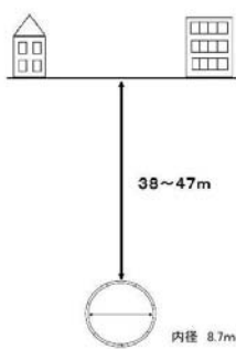
横断面図
