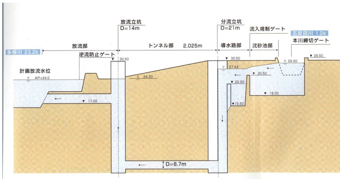
断面図
