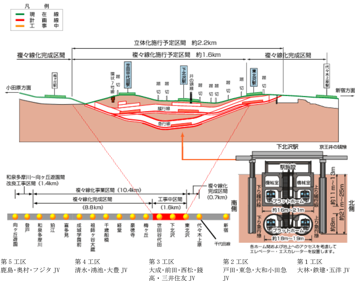
代々木上原～梅ヶ丘間の断面図
