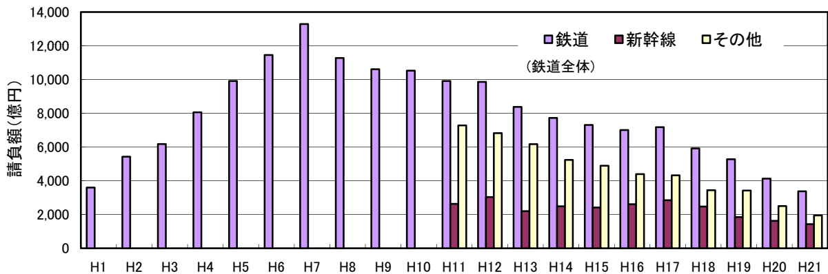
図-7 鉄道トンネルの推移
