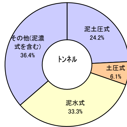
図-21 推進工法の形式比率
