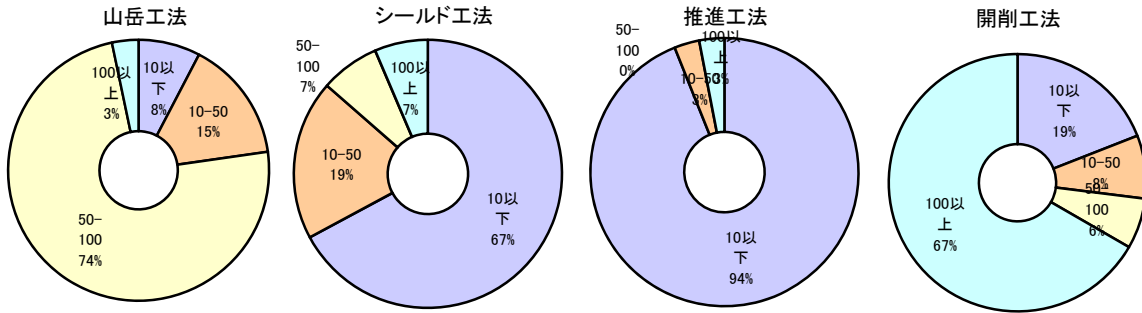
図-17 内空断面積(単位:m 2 )
