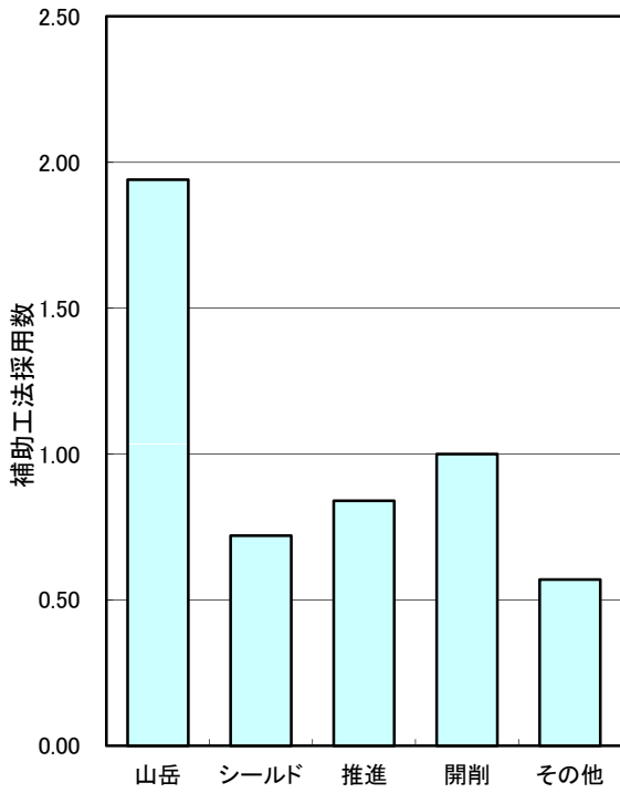
図-23 施工法と補助工法の採用数
