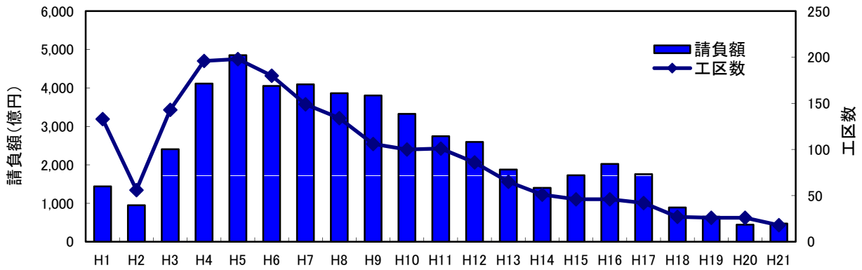
図-10 洞道管路の推移(専用洞道管路、共同溝等)
