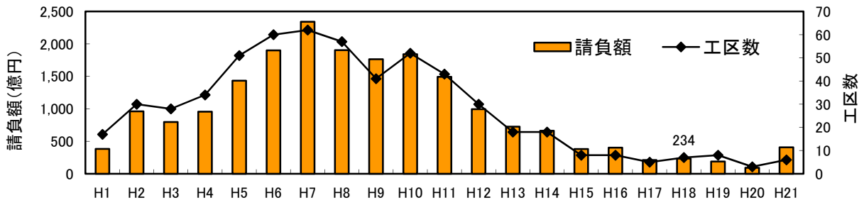
図-4 地下街・地下駐車場等工事の推移
