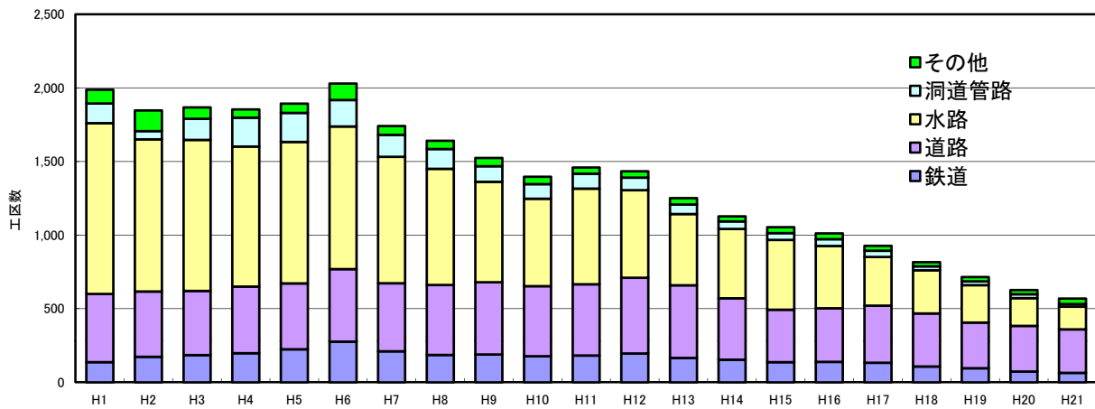
図-3 国内の工事量-工区数-の推移 (地下街を除く)
