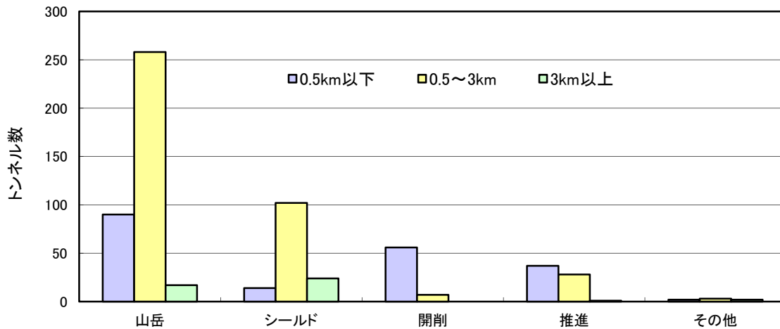
図-16 施工法と契約延長
