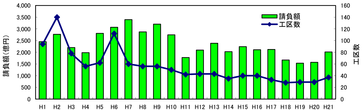
図-11 その他の推移(地下発関連、その他)
