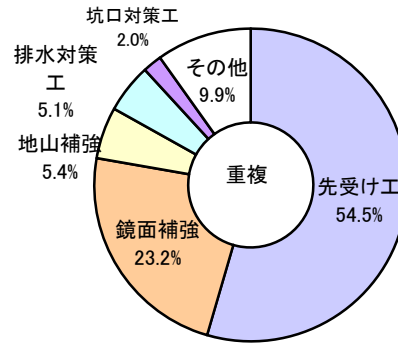
図-24 山岳工法における補助工法
