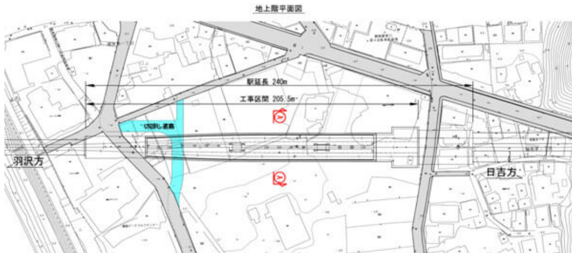
新網島駅(仮称)平面図・縦断図
