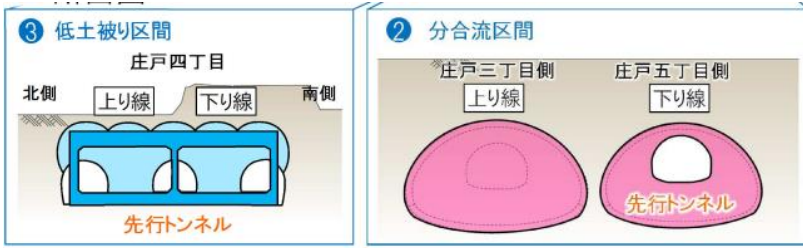
庄戸トンネル (パンフレットより)
