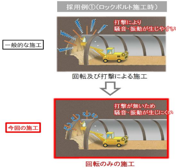
騒音・振動対策 (トンネル作業時) (パンフレットより)
