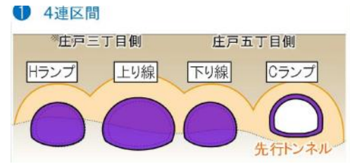
隣接の釜利谷西トンネル (パンフレットより)
