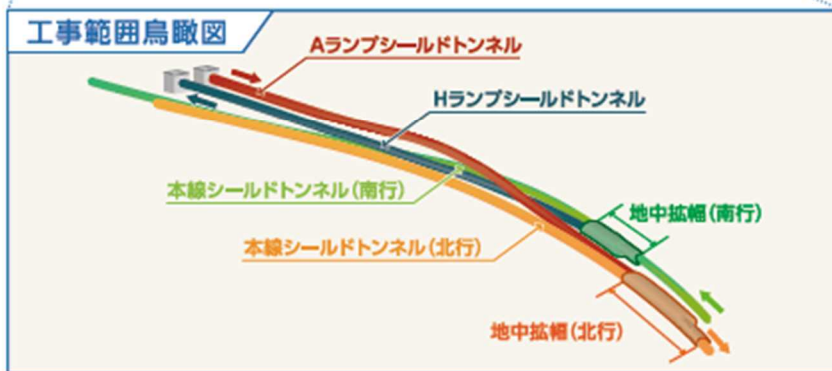
現場概要図
